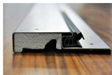
próg nierdzewny z wypełnieniem XPS
