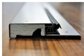
próg nierdzewny z wypełnieniem XPS
