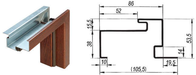
Ościeżnica FR Premium, asymetryczna z uszczelką (do drzwi metalowych PREMIUM WD, C, S)
