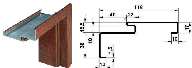
Ościeżnica FT SL, narożnikowa z uszczelką (do drzwi panelowych STANDARD WX10, CX10, SX10)
