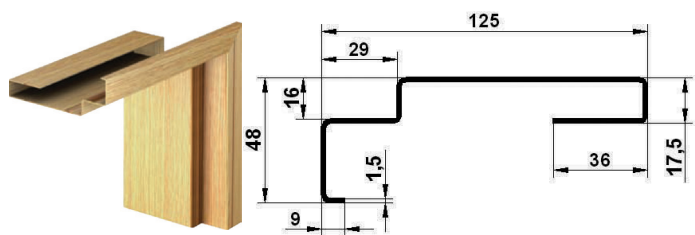
Ościeżnica FN, narożnikowa bez uszczelki (do drzwi metalowych STANDARD WD, C, S)
