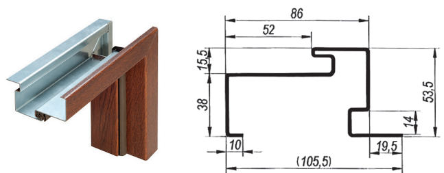
Ościeżnica FR Premium SL, asymetryczna z uszczelką (do drzwi panelowych PREMIUM WX10, CX10, SX10)
