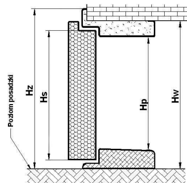
Rysunek poglądowy dla ościeżnic drzwi i progów dla: FN, FN SL
