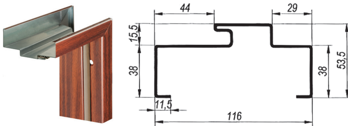
Ościeżnica FC Premium z uszczelką (do drzwi metalowych PREMIUM WD, C, S)
