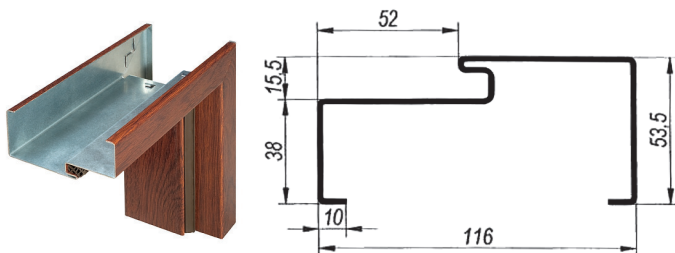
Ościeżnica FA Premium SL, asymetryczna z uszczelką (do drzwi panelowych PREMIUM WX10, CX10, SX10)
